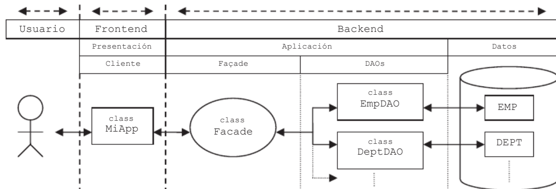
Fig. 8.2 Interacción entre el usuario, el frontend y el backend .
