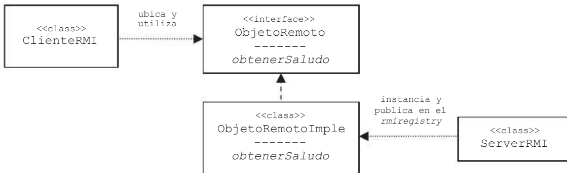
Fig. 7.1 Diagrama de clases de una aplicación RMI.
