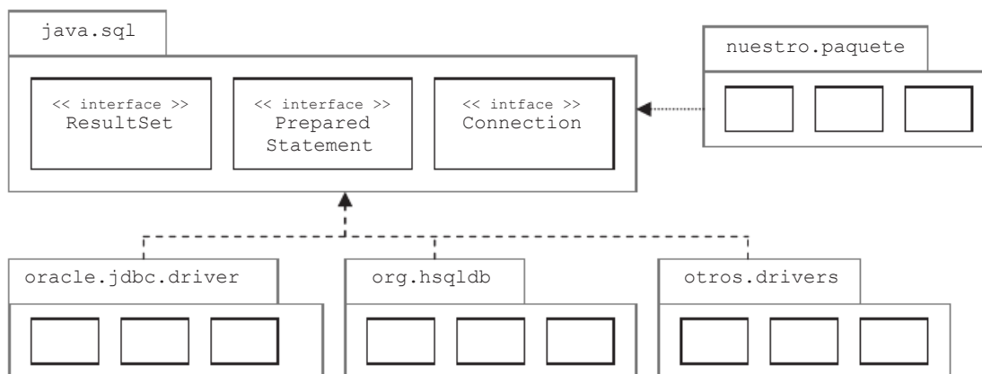
Fig. 3.2 Diagrama UML de dependencia de paquetes.
