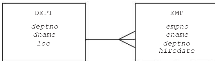
Fig. 3.1 Diagrama de Entidad/Relación.
