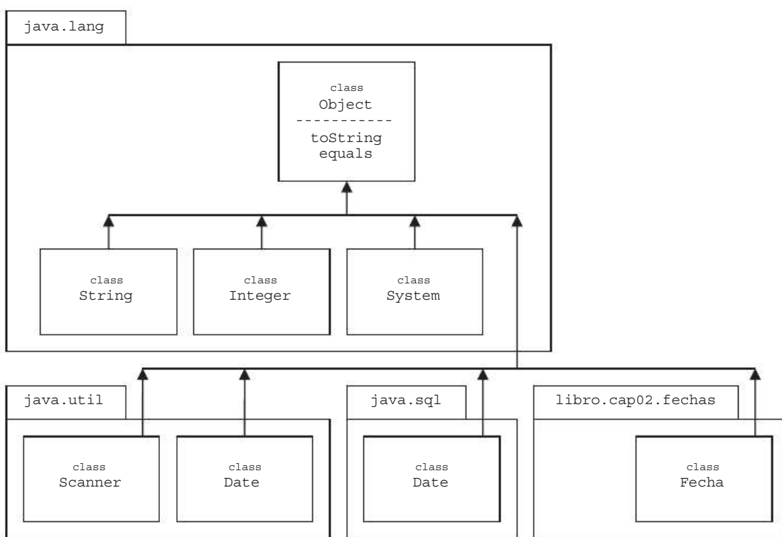
Fig. 2.1 Diagrama de clases y paquetes de UML.
