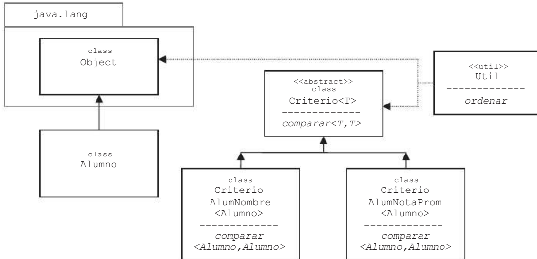
Fig. 2.5 Implementaciones de la clase Criterio<T>.
