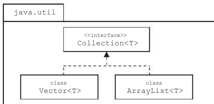
Fig. 2.6 Representación de las clases Vector y ArrayList
