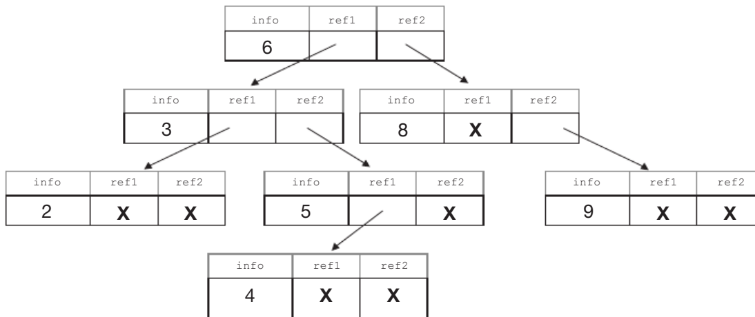
Fig. 9.5 Árbol binario.
