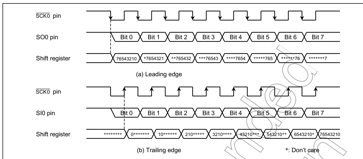
Figure 2.10.20 Shift Edge
