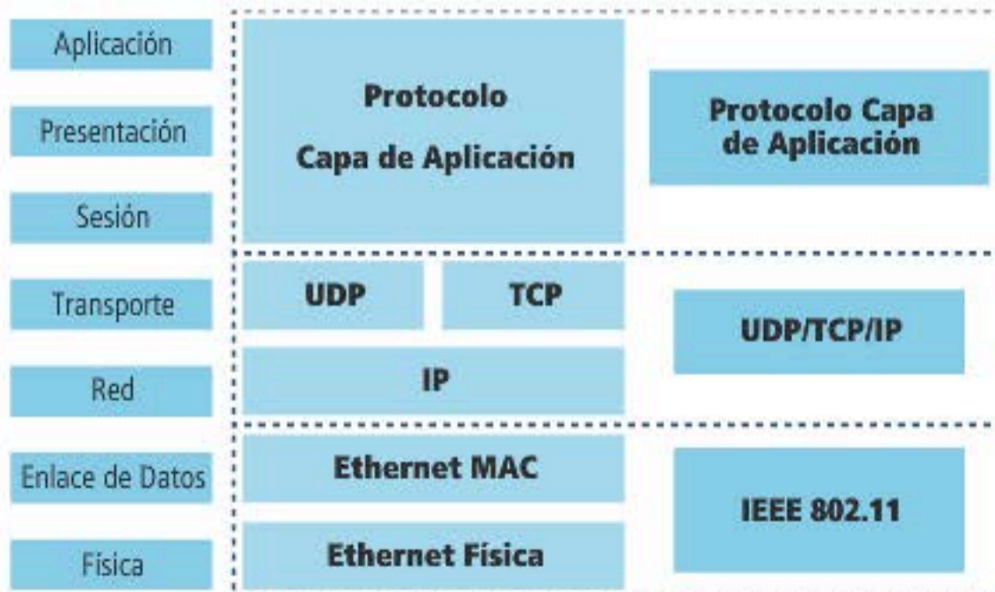
Capas de injerencia del estándar 802.11 en el modelo OSI. Podemos ver claramente que se ubica en la capa física y la subcapa MAC.
