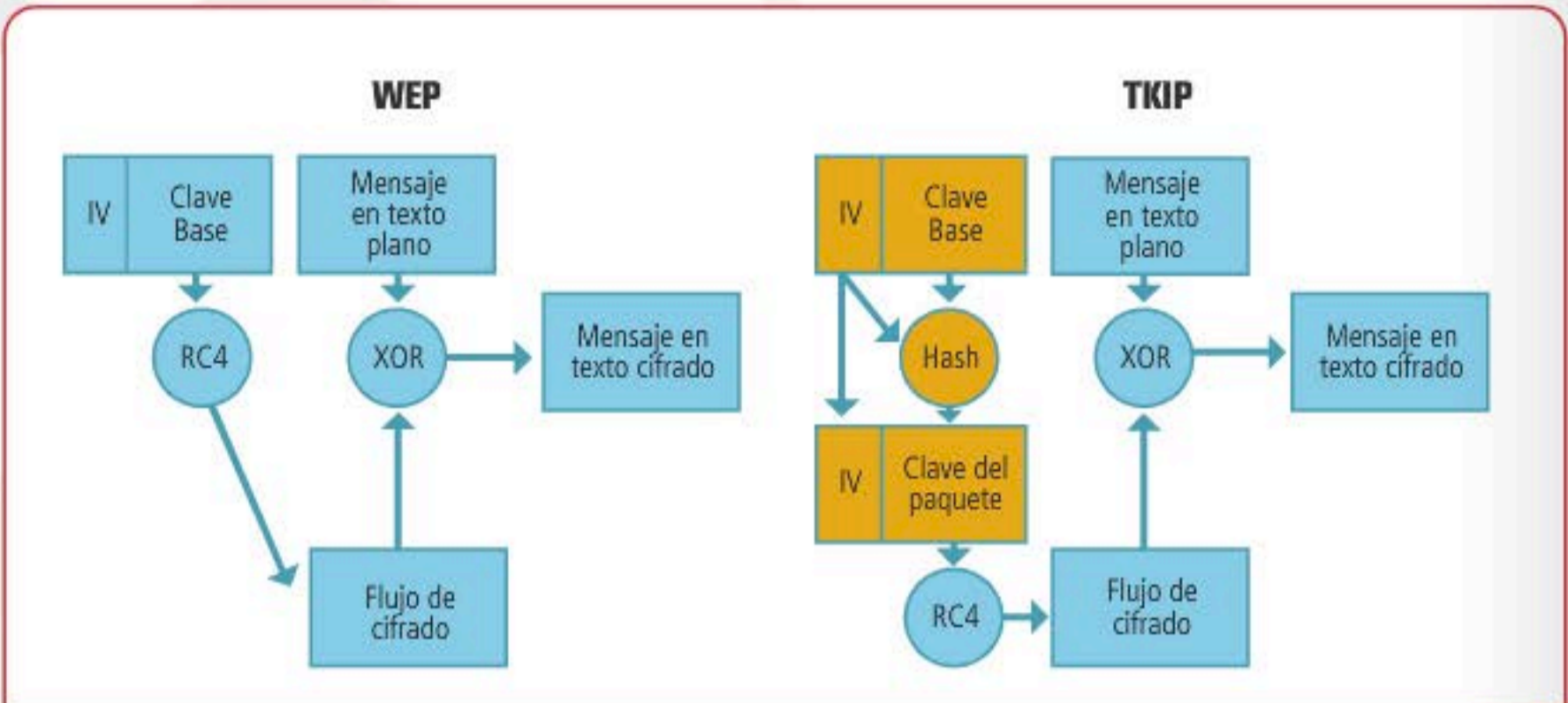
En este diagrama, podemos apreciar que WEP usa un IV y una clave base que genera IVs débiles. TKIP usa IV y clave base para producir un hash que será la nueva clave, distinta por paquete.
