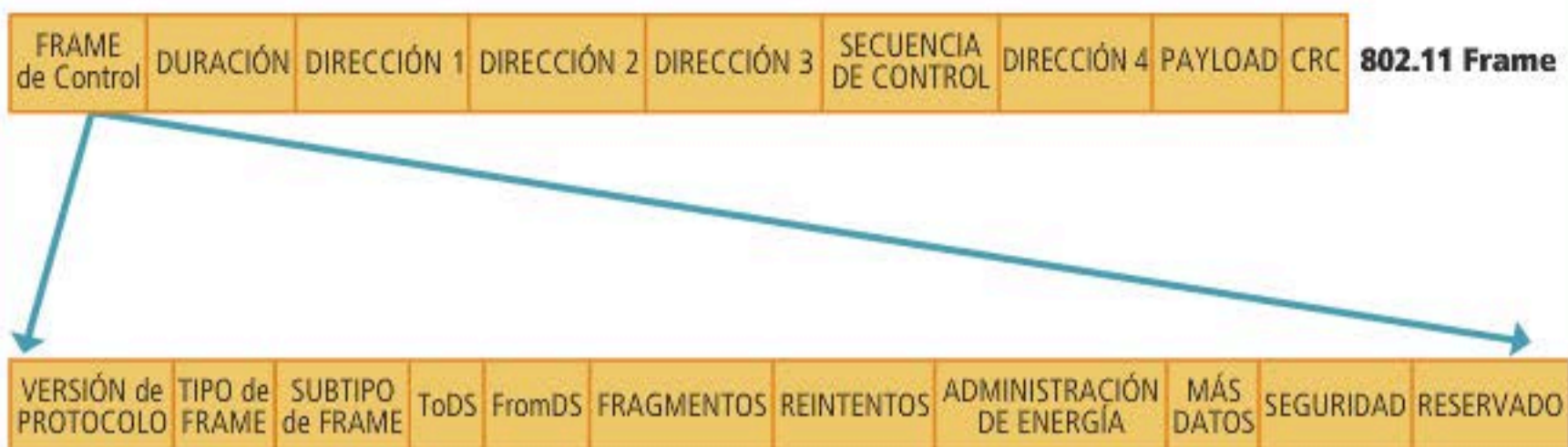
Diagrama que muestra la composición del frame o trama en el estándar 802.11.
