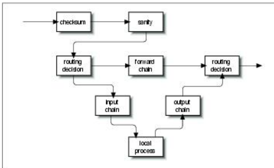
Figura 9-9. Cadena de procesamientos de datagramas en 'netfilter'
